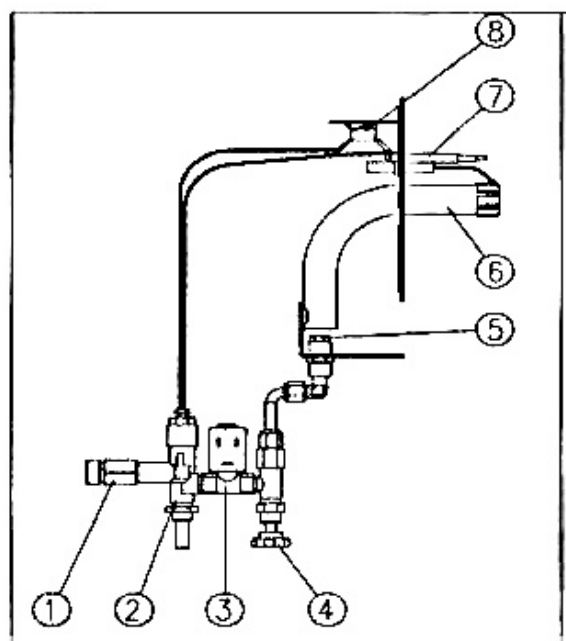
1. Przyłącze gazu, 2. Zawór, 3. Zawór elektromagnetyczny, 4. Zawór, 5. Czujnik płomienia, 6. Igła zapłonowa, 7. Termostat, 8. Głowica palnika
