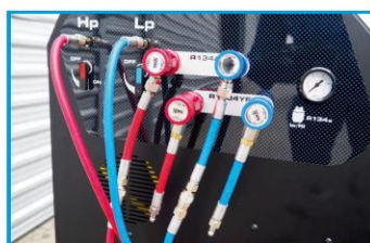
DVOJITÝ SYSTÉM SPOJOK R134a A HFO1234yf
