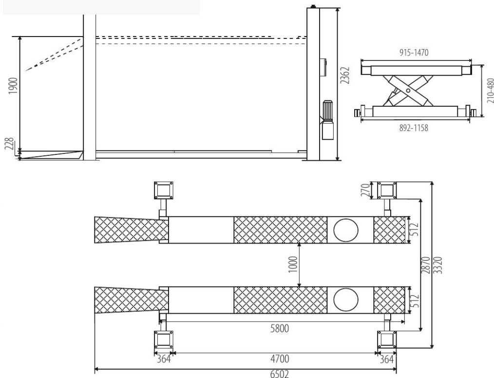
ZDVIHÁK NÁPRAVY 3,2 T S PNEUMATICKÝM ČERPADLOM
